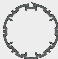
Rullo maggiorato diametro 48 mm Ø interno 41,50 mm Ø esterno 49,10 mm
