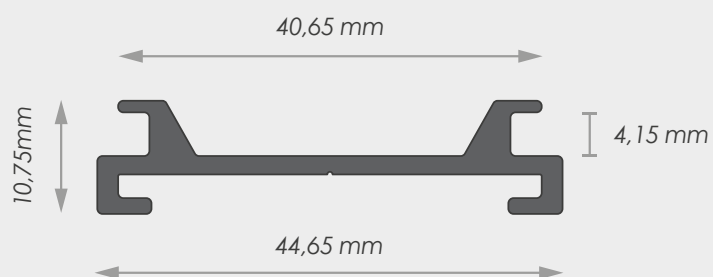
Guida superiore (bianco o argento ossidato)
